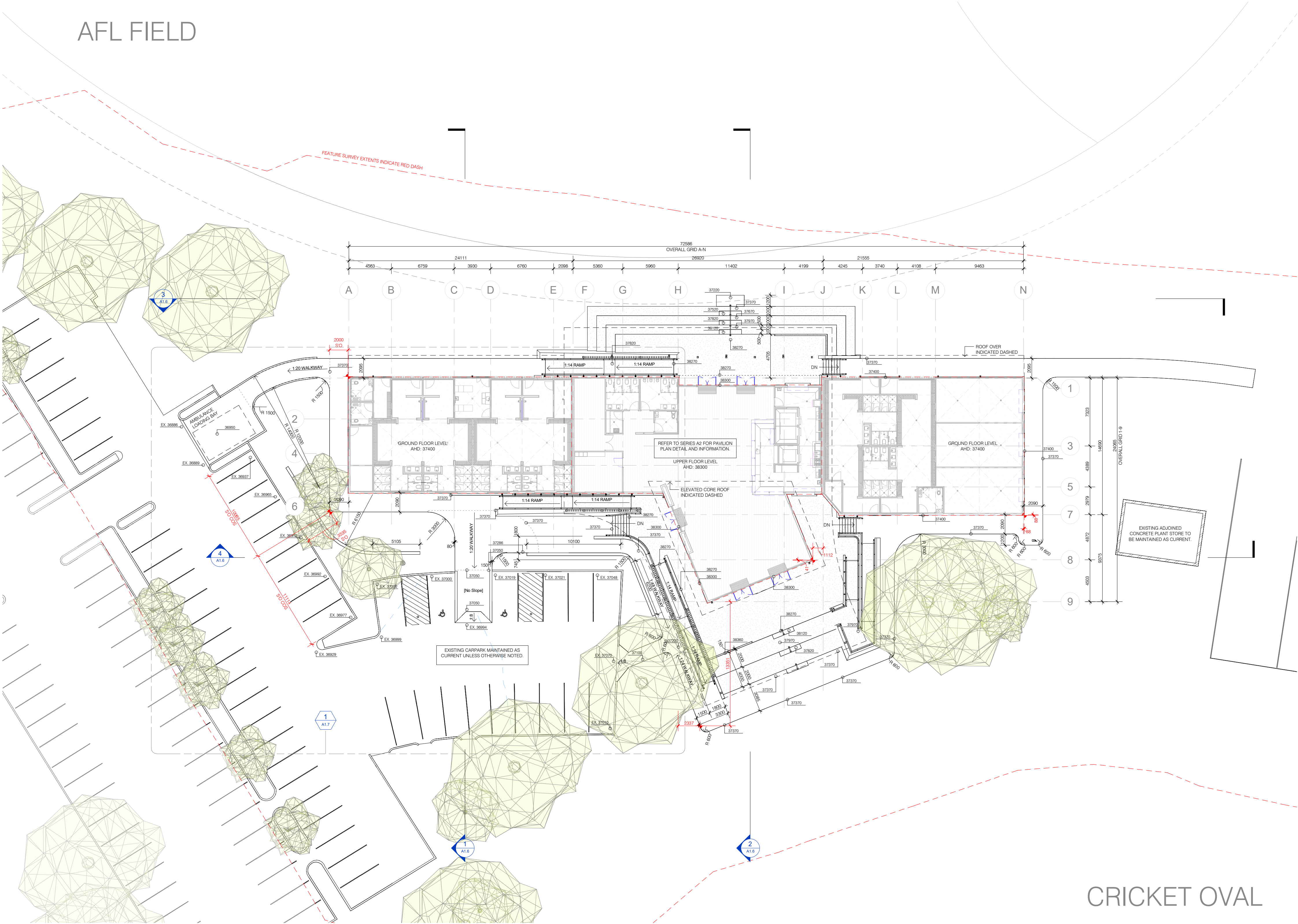
1 SA - PAVILION LAYOUT PLAN A1.6 1 : 200
