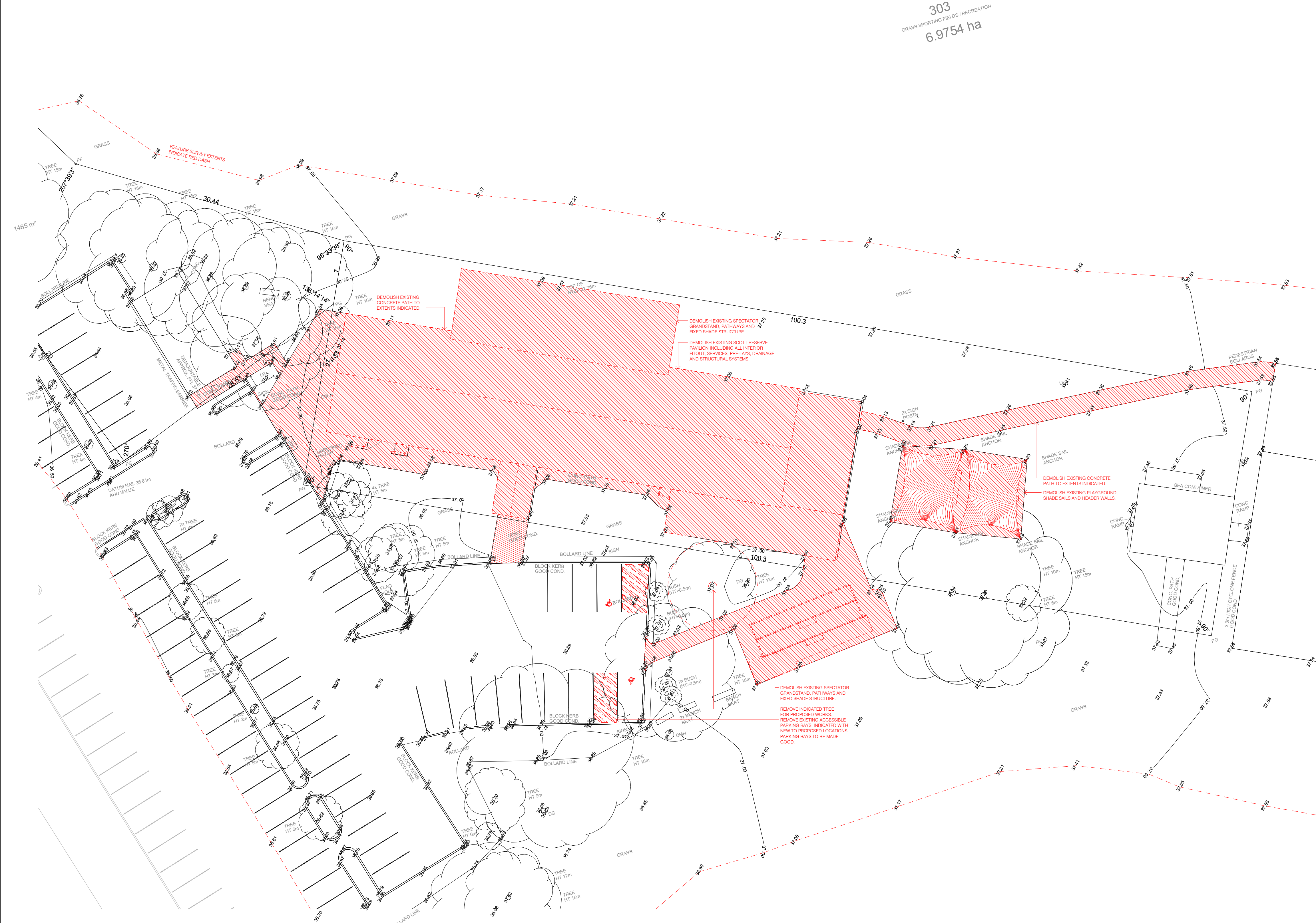
1 SA - DEMOLITION PLAN 1 : 200
